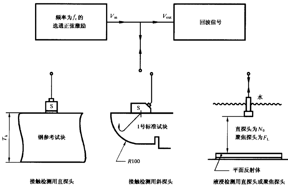
接触检测用直探头
