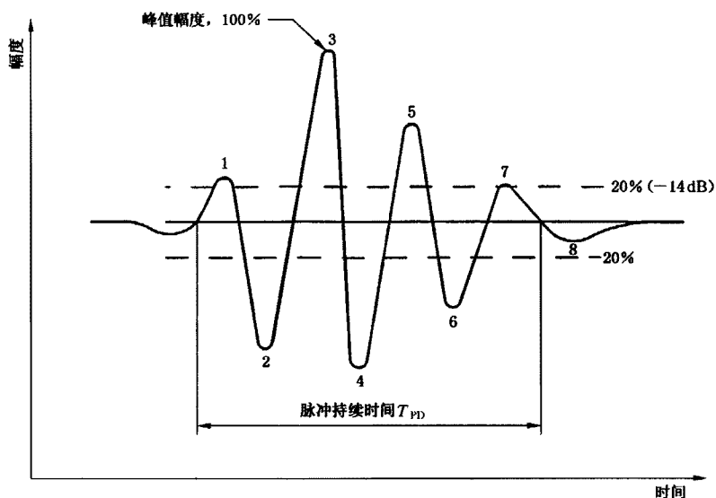
图 5 时域响应
