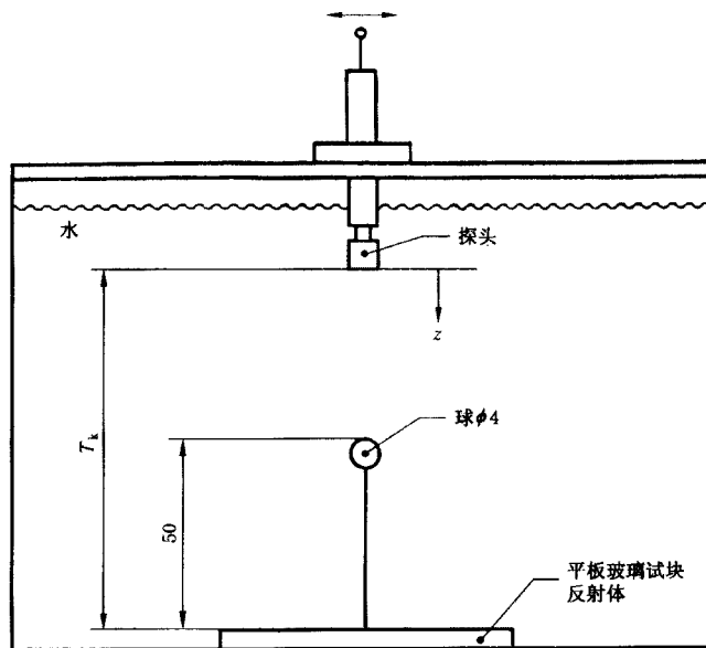
图 1 采用电冲击激励的超声脉冲反射法检测的测试装置
