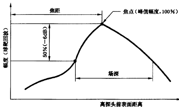
图 10 液浸聚焦探头声束轴线上的声压分布
