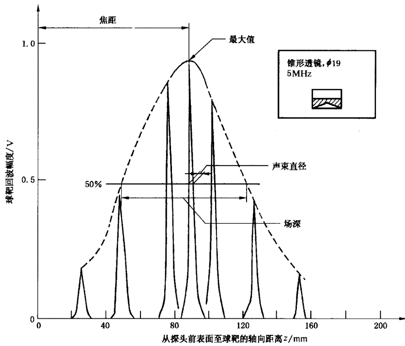
图 11 液浸聚束探头声束轴线上和横截面声压分布和声束直径
