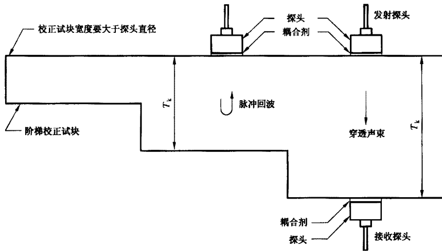
图3 直探头接触检测的测试布置
