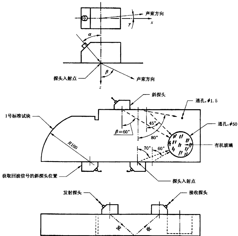
图4 斜探头接触检测的测试布置
